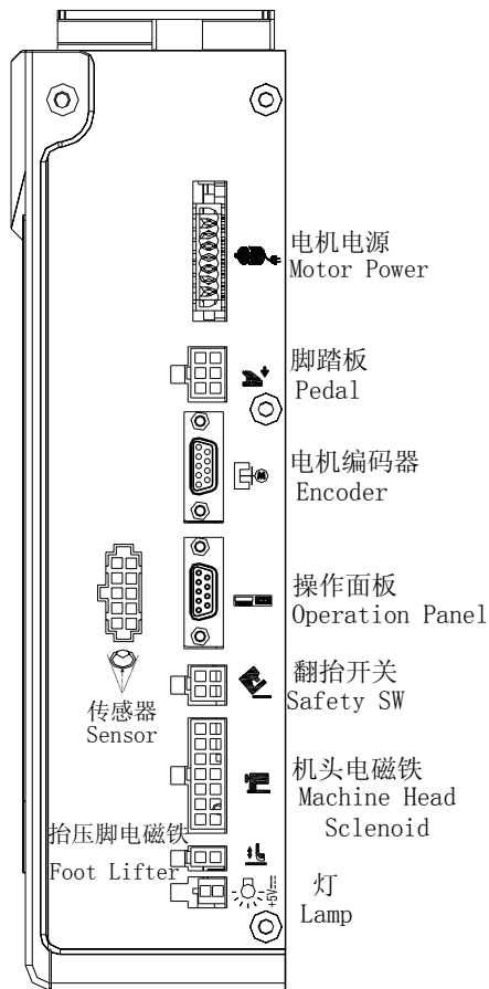
图 3-1 控制器对外接口示意图
